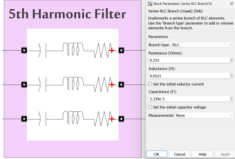
شكل 6: نافذة بارامترات مرشح التوافقية الخامسة في ماتلاب
